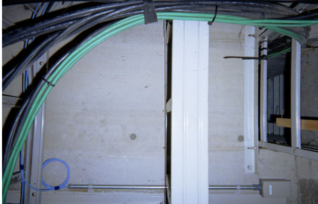
地下共同溝内ケーブル設置
